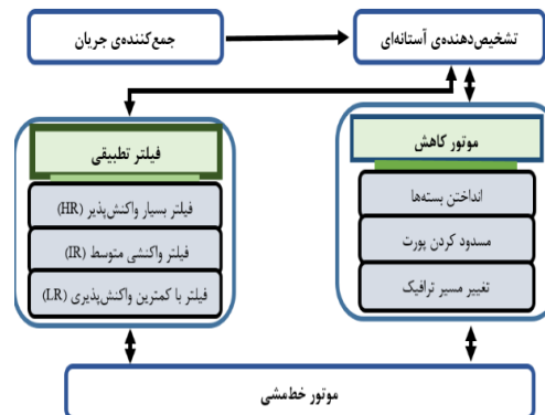
(شکل-۹): طرح چارچوب دفاعی پیش فعال [۱۱]
