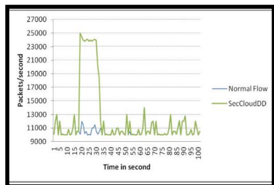
(شکل-۱۲): تشخیص حمله DDOS به روش
