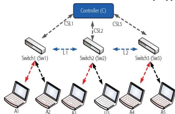
(شکل-۶): توپولوژی SDN در برابر تهدیدات DDoS [۲۰]
