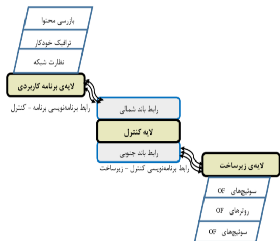
(شکل-۱): اجزاء و معماری سه‌لایه‌ای SDN [۱۶]
