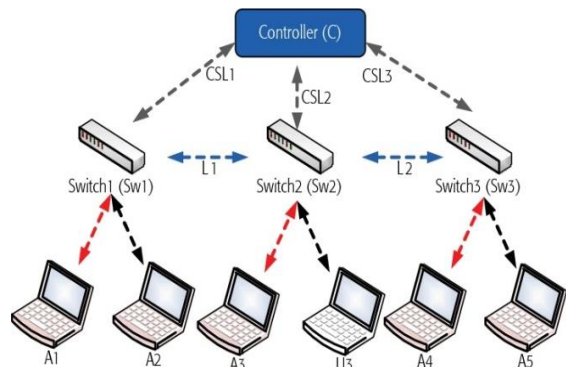
(شکل-۶): توپولوژی در برابر تهدیدات DDos [۲۰]
