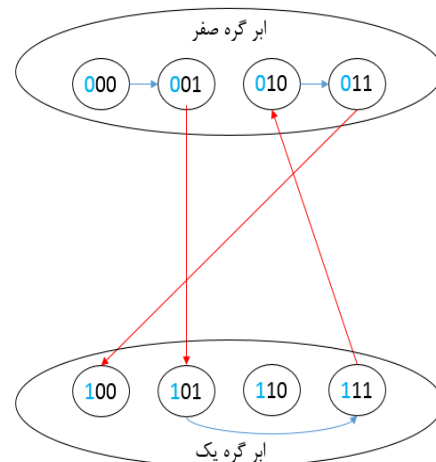
(شکل ۴): نمایش گرافیکی تابع اسفنجی با r=2 و c=1
